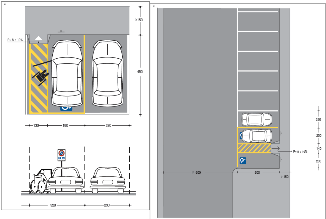
Figura II 445/a Art. 149 DELIMITAZIONE DEGLI STALLI DI SOSTA RISERVATI AGLI INVALIDI (dimensioni in centimetri)
